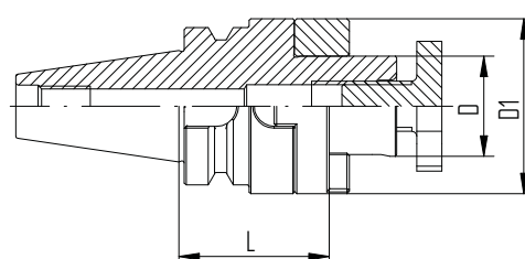
Croquis 2 BT/KFD
