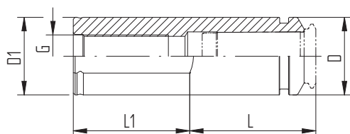
Dessin 5
