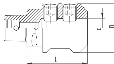
Croquis 2 C/WD
