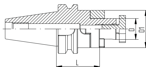
Croquis 1 BT/KFD
