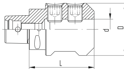
Croquis 2 C/WD
